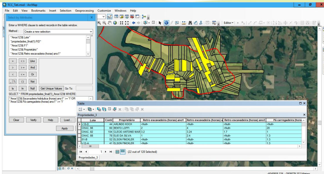
Figura 6. Ferramenta de consultas SQL.
