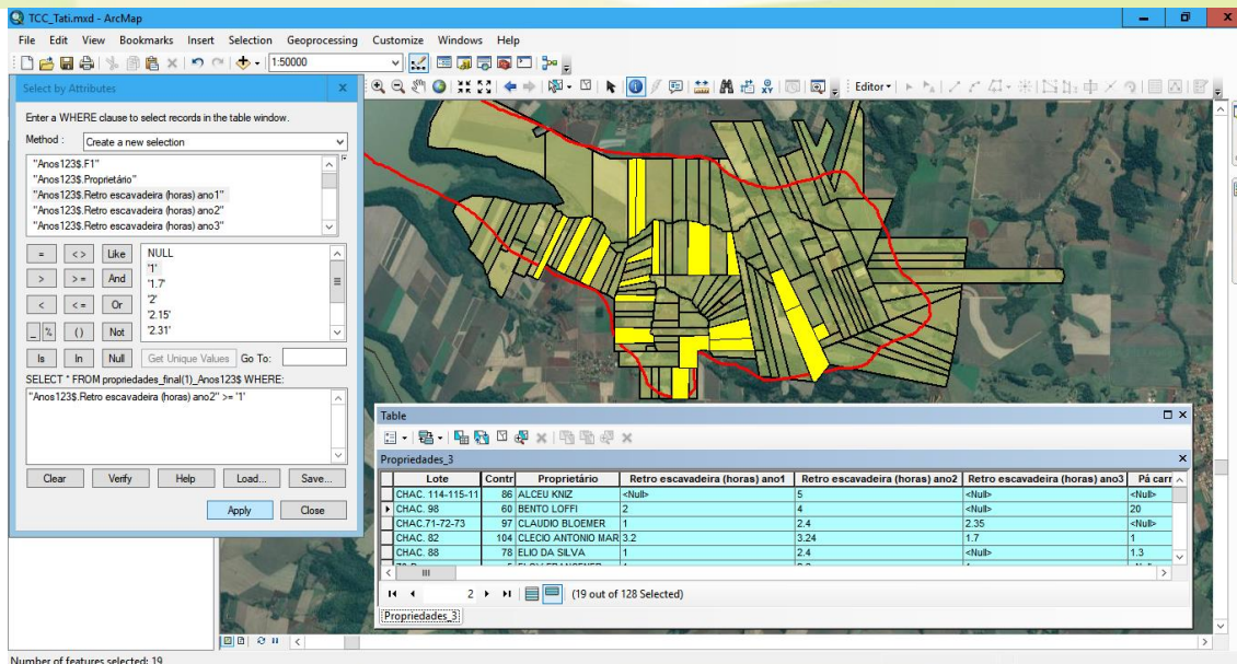
Figura 14. Consulta SQL- Localização de propriedades que receberam horas de retro escavadeira no ano 2 (2016).
