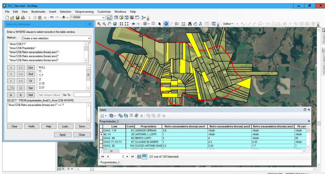
Figura 13. Consulta SQL- Localização de propriedades que receberam horas de retro escavadeira no ano 1 (2015).
