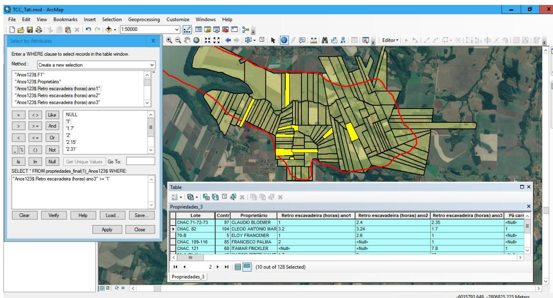
Figura 15. Consulta SQL- Localização de propriedades que receberam horas de retro escavadeira no ano 3 (2017).
